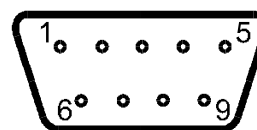
Rys. 1-16 ZŁĄCZE WAGI
