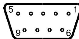
Rys. 1-13 ŁĄCZE PC
