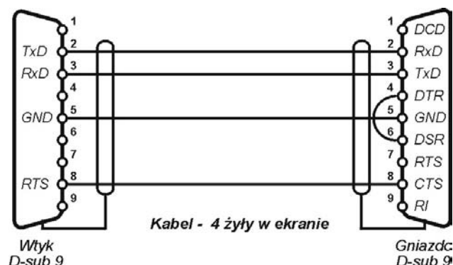
Rys. 1-18 Schemat połączeń wewnętrznego kabla do komputera
