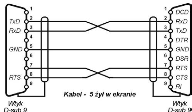
Rys. 1-19 Schemat połączeń wewnętrznego kabla do kasy
