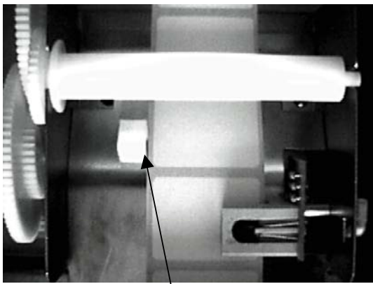
Rys. 1-8 Kołek blokujący w punkcie A oraz widok w zbliżeniu
