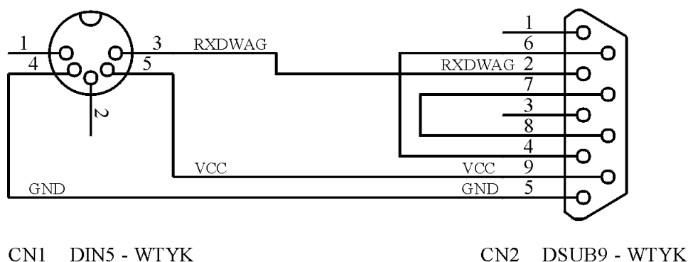
Rys. 1-20 Przejściówka szeregowego czytnika kodów kreskowych.
