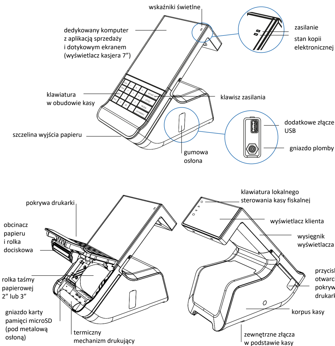
Rozmieszczenie elementów kasy
